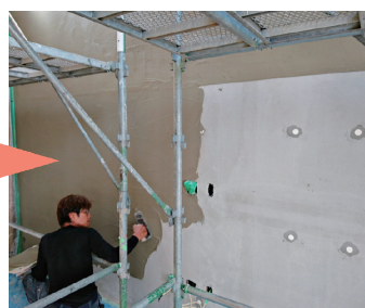
最終下地 塗り厚:3mm
