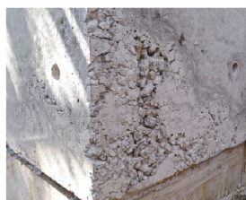
ジャンカ、アバタ
